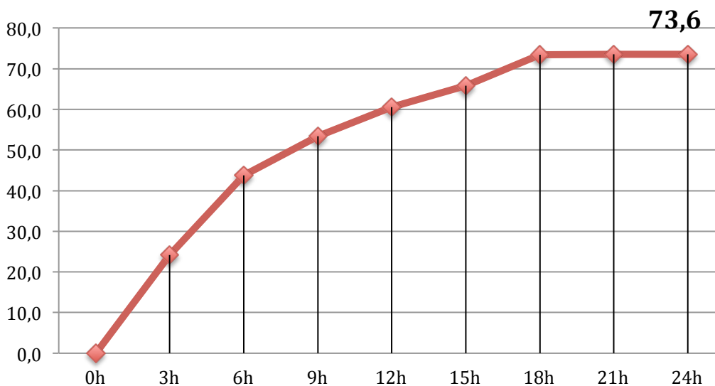
Evolución lluvia acumulada en BARXETA el día 15 en períodos de 3 horas (en l/m 2 )
