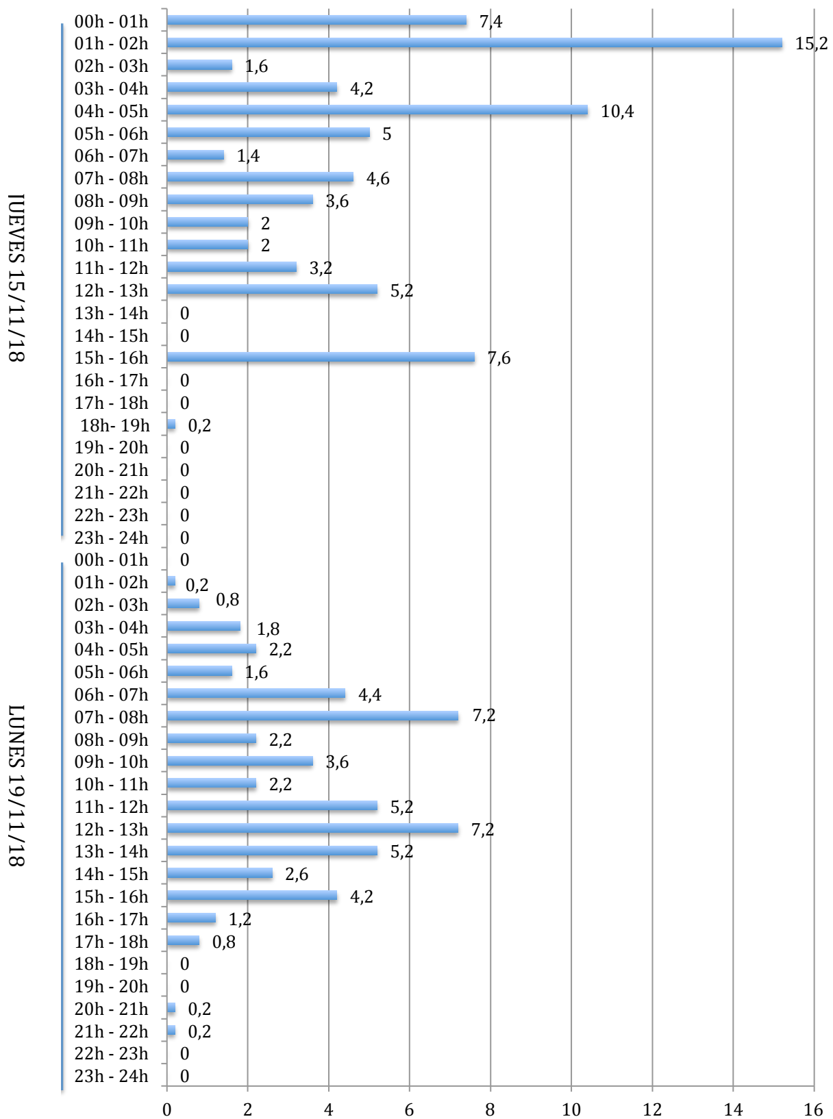
Cantidades de lluvia registradas por horas en BARXETA los días 15 y 19/11/18 (en l/m 2 )
