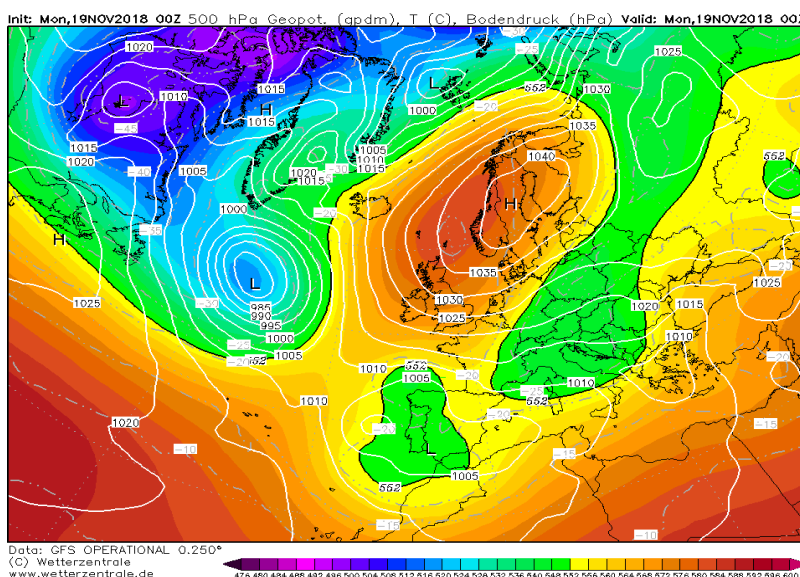
Situación sinóptica de los días 18 y 19 de Noviembre de 2018 (00Z) Geopotencial a 500hPa y mapa de superficie
