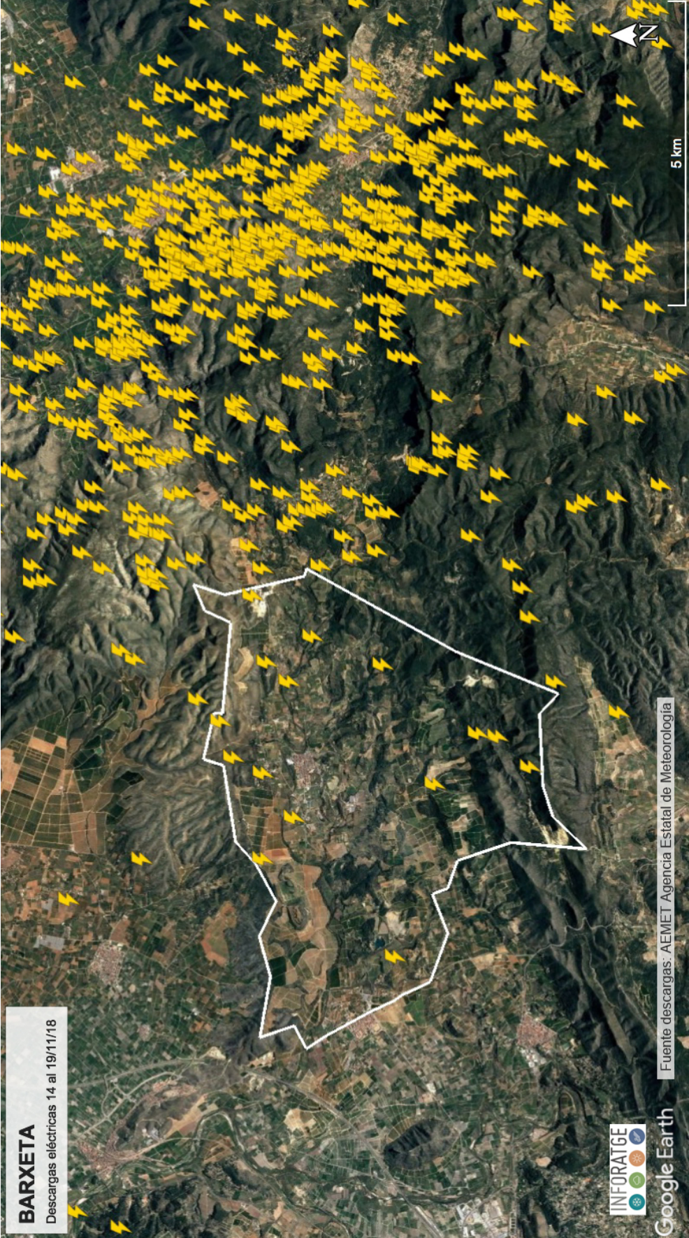
Geolocalización de las descargas eléctricas “nube-tierra” registradas en el término municipal de BARXETA y alrededores entre los días 14 y 19/11/18
